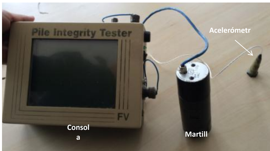
Figura 2. Equipo utilizado para las pruebas PIT.
